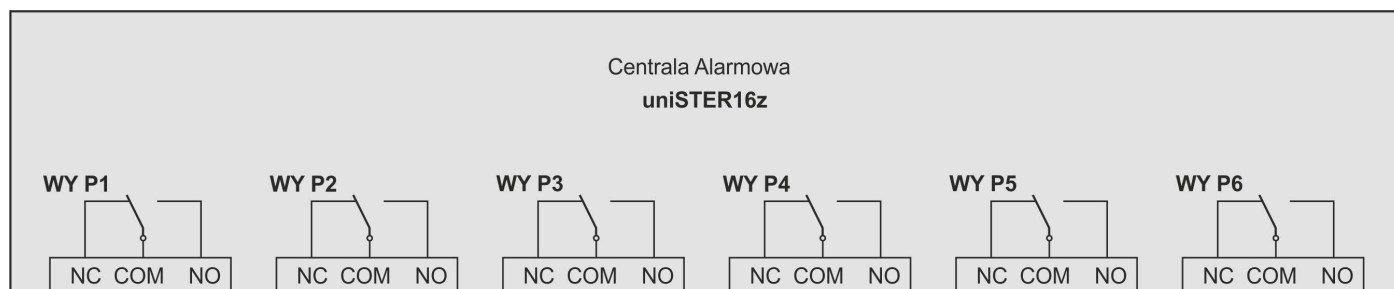
Rys.4. Schemat wyjść stykowych (przekaźnikowych) Centrali Alarmowej uniSTER16z
