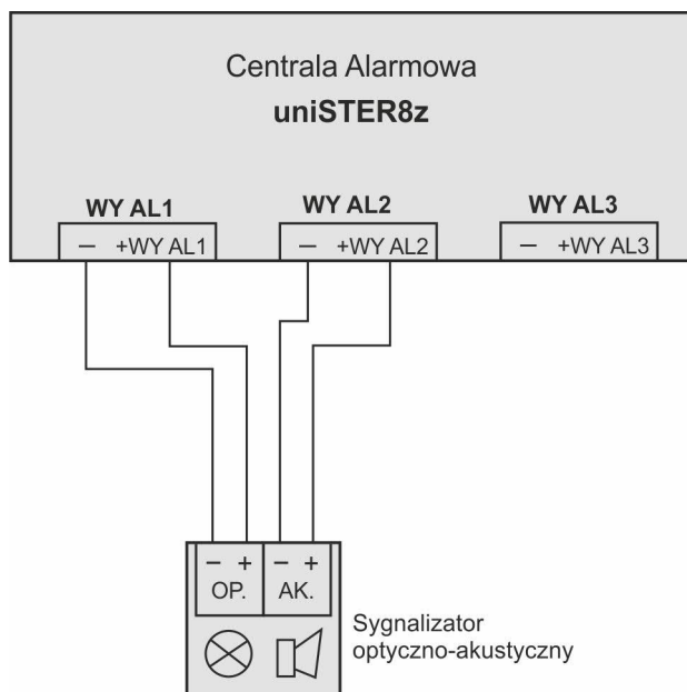
Rys.5. Podłączenie sygnalizatora optyczno-akustycznego z Centralą Alarmową uniSTER8z
