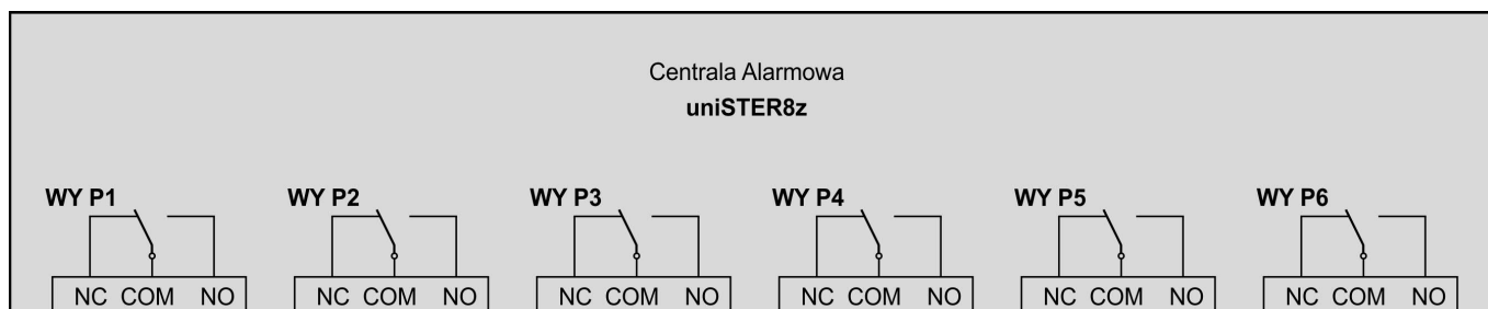
Rys.4. Schemat wyjść stykowych (przekaźnikowych) Centrali Alarmowej uniSTER 8z
