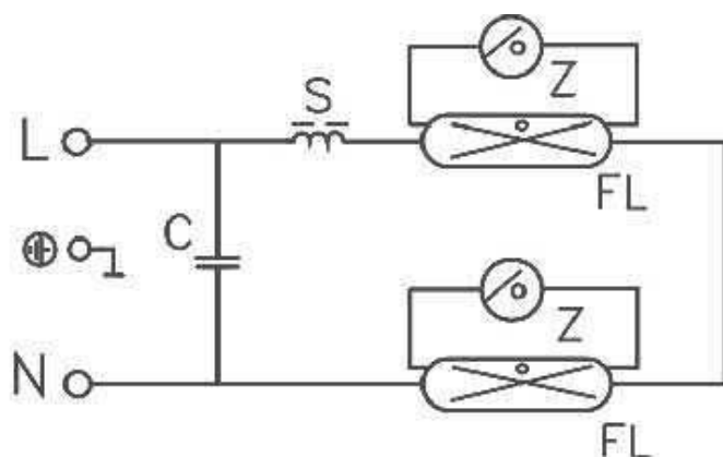
Rys.2. Schemat połączeń elektrycznych lampy AWF-18 (AWF-18Z)
