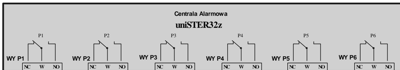
Rys.5. Schemat wyjść stykowych (przekaźnikowych ) Centrali Alarmowej uniSTER32z
