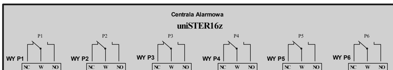
Rys.4. Schemat wyjść stykowych (przekaźnikowych ) Centrali Alarmowej uniSTER16z
