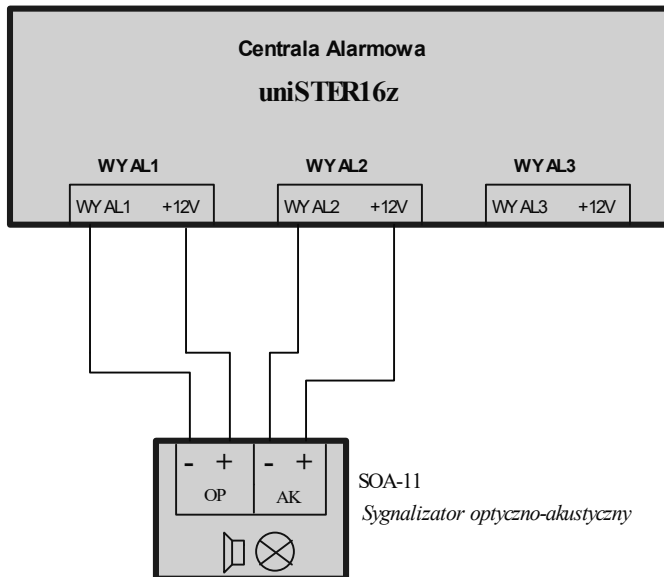
Rys.5. Podłączenie sygnalizatora optyczno-akustycznego z Centralą Alarmową uniSTER16z
