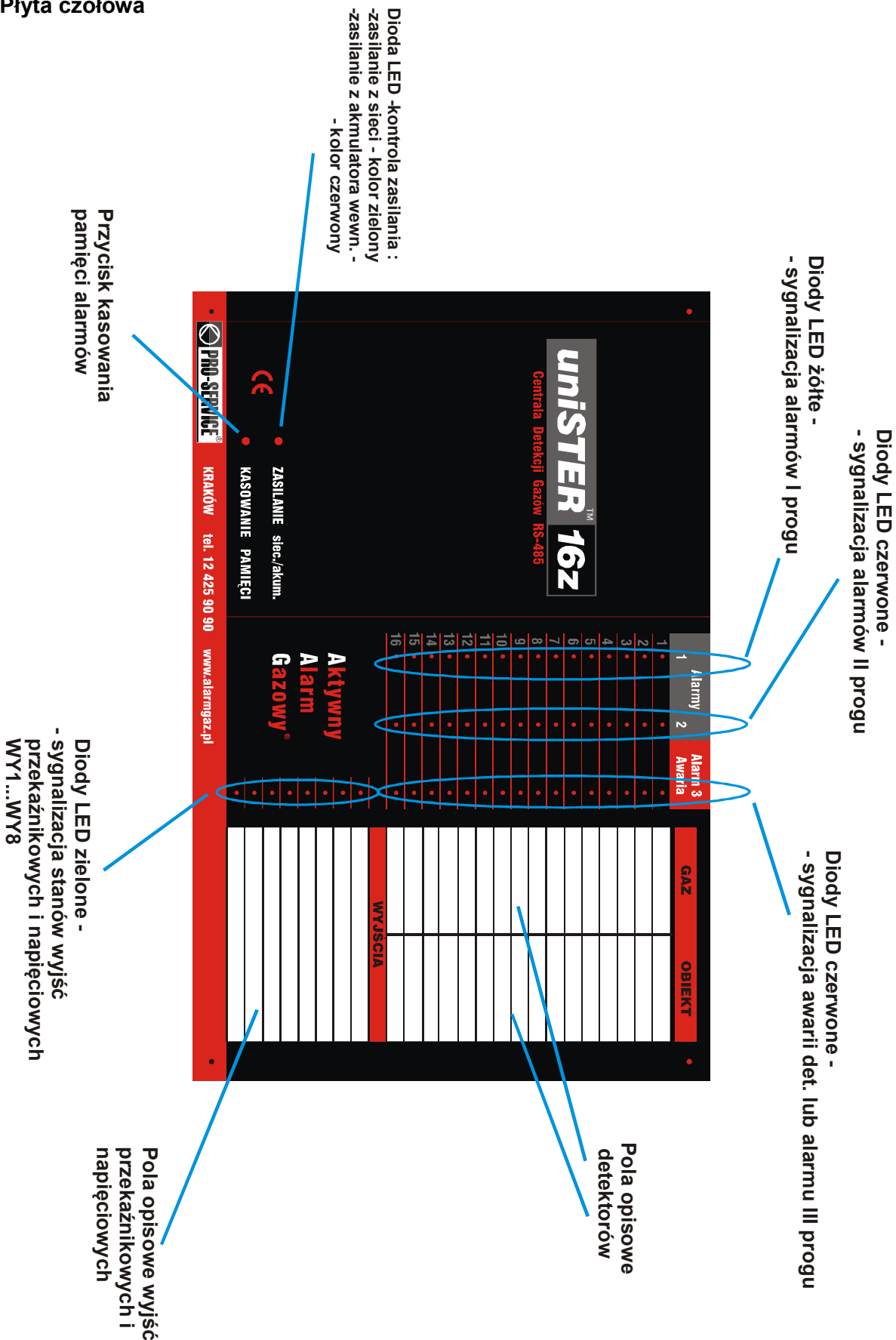
Rys.1. . Płyta czołowa Centrali Alarmowej „uniSTER 16z/RS485”
