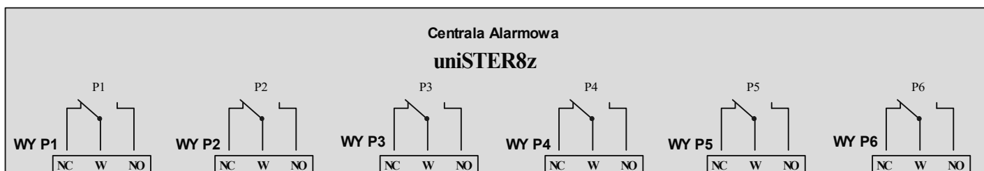
Rys.4. Schemat wyjść stykowych (przekaźnikowych ) Centrali Alarmowej uniSTER 8z
