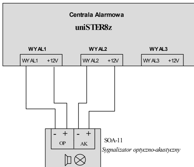
Rys.5. Podłączenie sygnalizatora optyczno-akustycznego SOA-11 z Centralą Alarmową uniSTER8z
