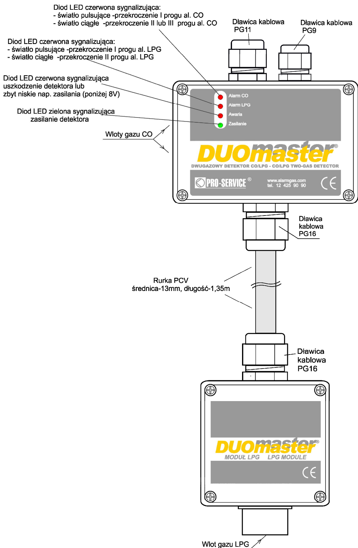
Rys.1. Widok Dwugazowego Garażowego Detektora „DUOmaster CO/LPG G”
