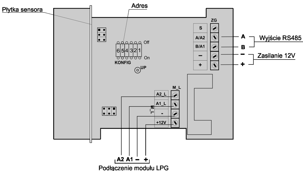
Rys.2. DUOmaster CO/LPG G –listwy zaciskowe modułu głównego
