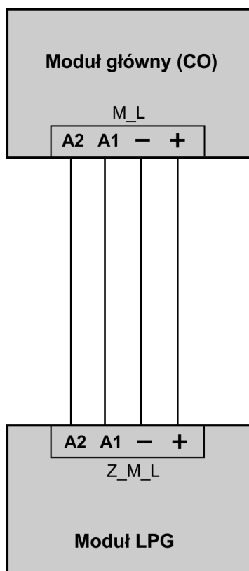
Rys.4. DUOmaster CO/LPG G –połączenie modułu głównego i modułu LPG
