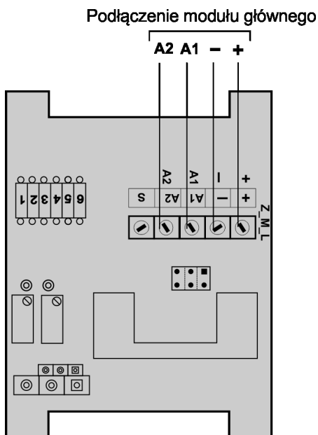
Rys.3. DUOmaster CO/LPG G –listwa zaciskowa modułu LPG
