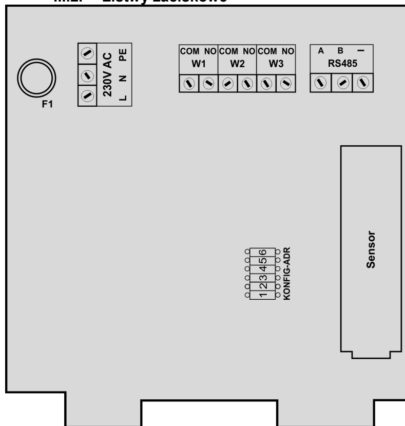
Rys.2. Listwy zaciskowe
