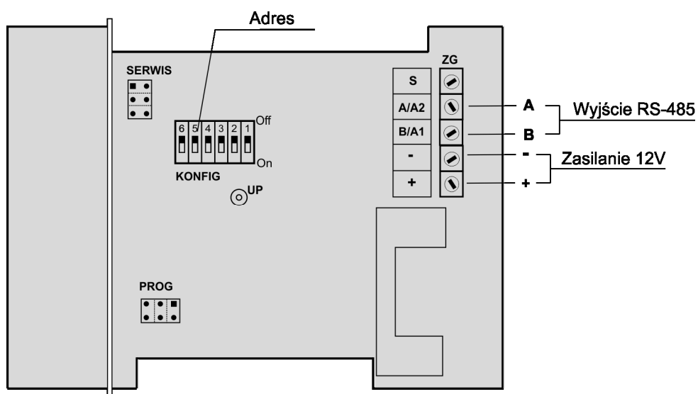
Rys.2. Listwa zaciskowa Detektora Tlenku Węgla „uniTOX.CO G /RS485” .
