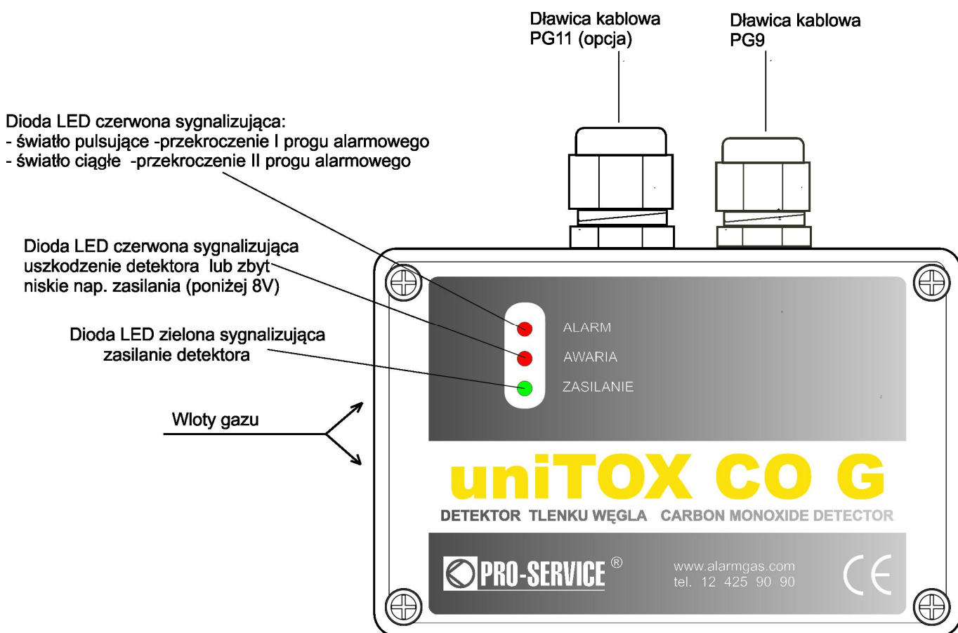
Rys.1. Widok Detektora Tlenku Węgla „uniTOX.CO G /RS485”
