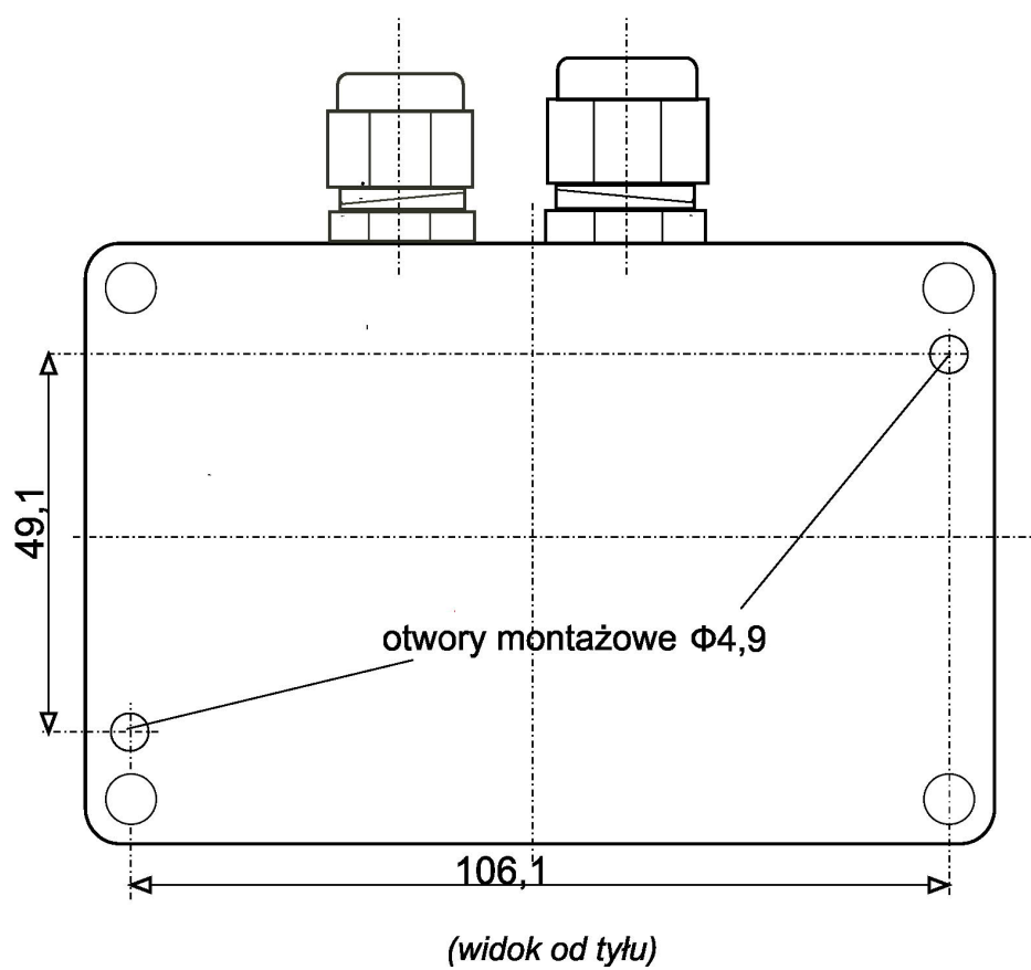
Rys.3. Wymiary Detektora Tlenku Węgla „uniTOX.CO G /RS485” .
