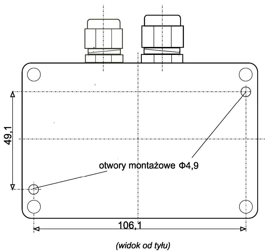
Rys.3. Wymiary Detektora Tlenku Węgla „uniTOX.CO G /RS485” .
